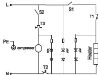
Электрическая схема
